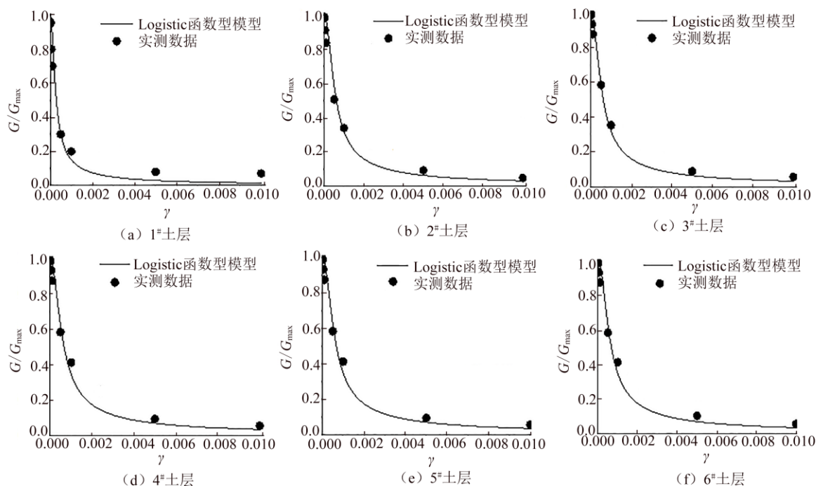
图6 动剪切模量比验证结果
