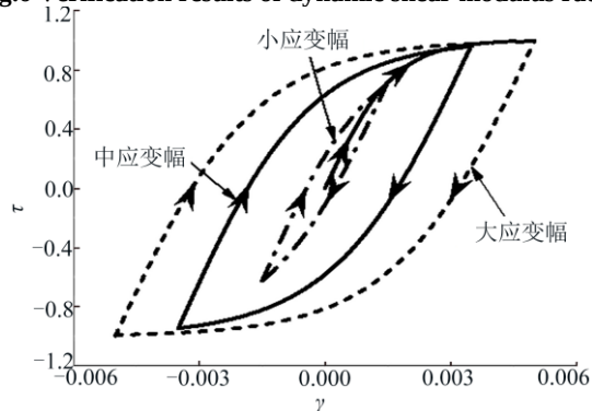
图7 不同应变水平下滞回曲线
